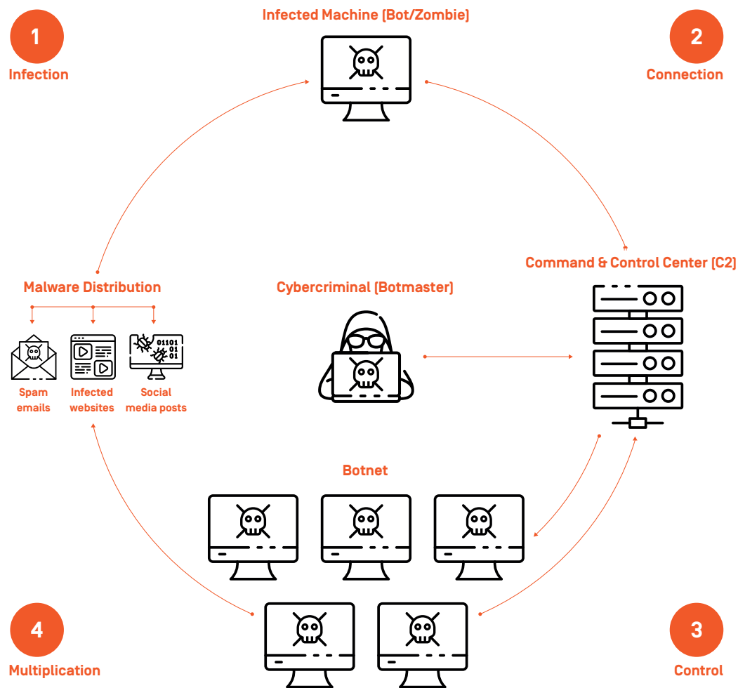
Figura I-3: Representação gráfica do funcionamento de uma Botnet
